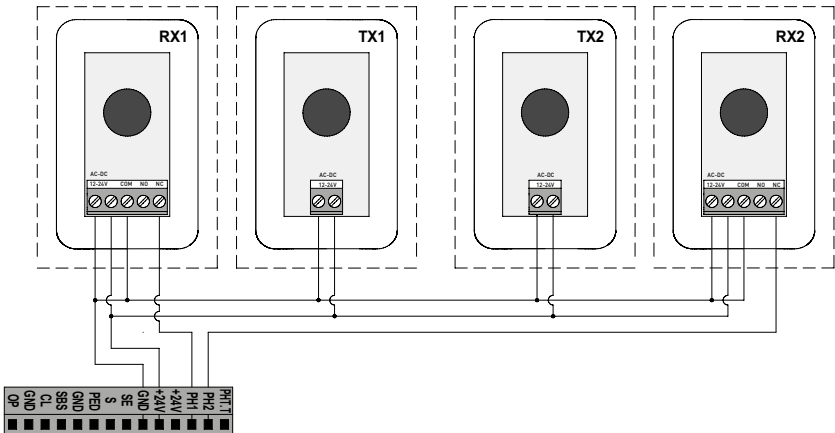
Малюнок 12. Схема підключення фотоелементів
