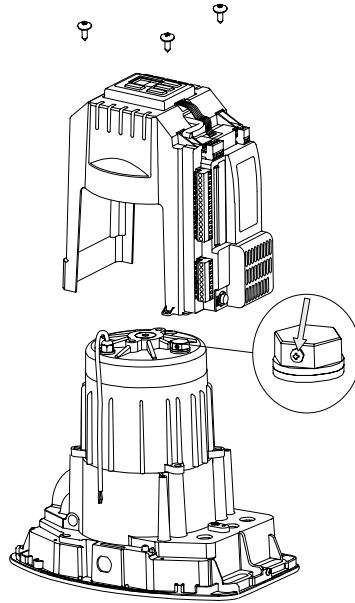
Малюнок 7. Гвинт сапуна на двигуні RTO-2000
