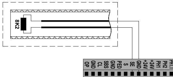
Малюнок 14. Схема підключення резистивної кромки безпеки 8,2 кОм
