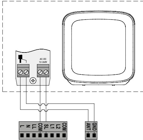
Малюнок 15. Схема підключення сигнальної лампи
