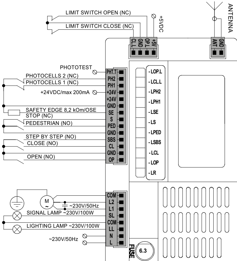
Малюнок 11. Електронний модуль керування
