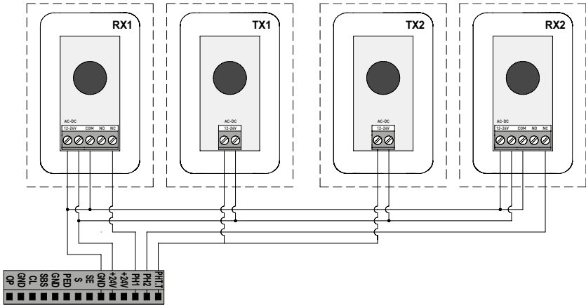
Малюнок 13. Схема підключення фотоелементів для роботи в режимі «фототест»
