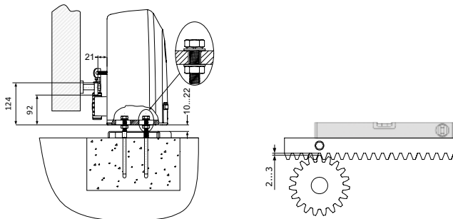
Малюнок 5. Регулювання положення двигуна
