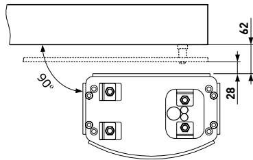
Малюнок 4. Розташування монтажної основи відносно до стулки
