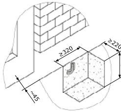
Малюнок 2. Підготовка під фундамент
