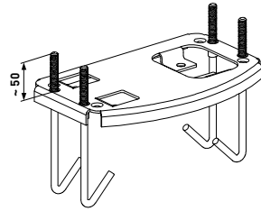
Малюнок 3. Монтажна основа
