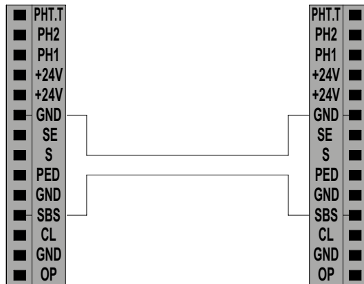
Малюнок 16. Схема підключення двох електронних блоків керування для синхронізації роботи двох двигунів
