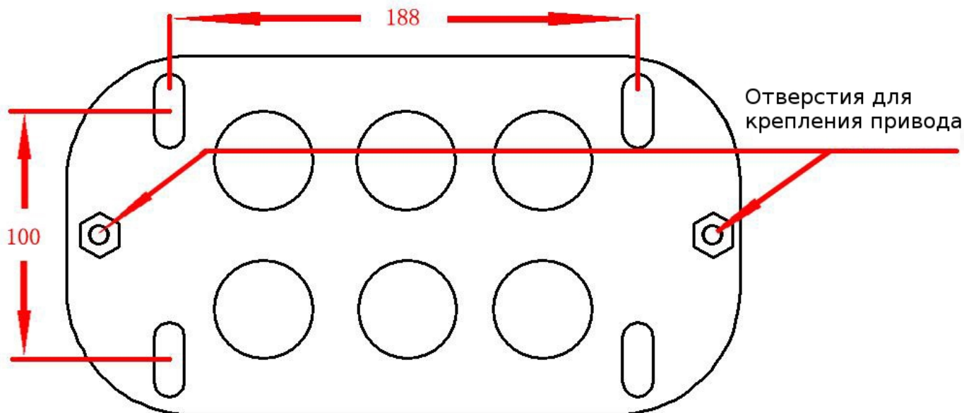
Рис. 2 Размеры монтажной пластины привода
