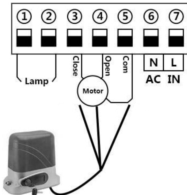
Рис. 9. Подключение электропривода к плате управления
