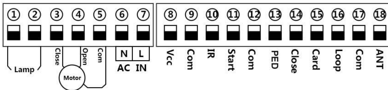
Рис. 8. Подключение питания привода
